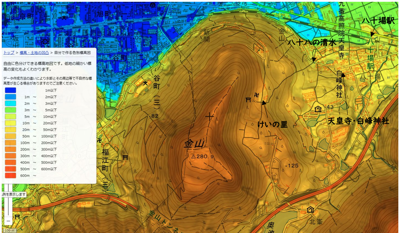
坂出市金山周辺の地形 (国土地理院地理地図・自分で作る色別標高図)
